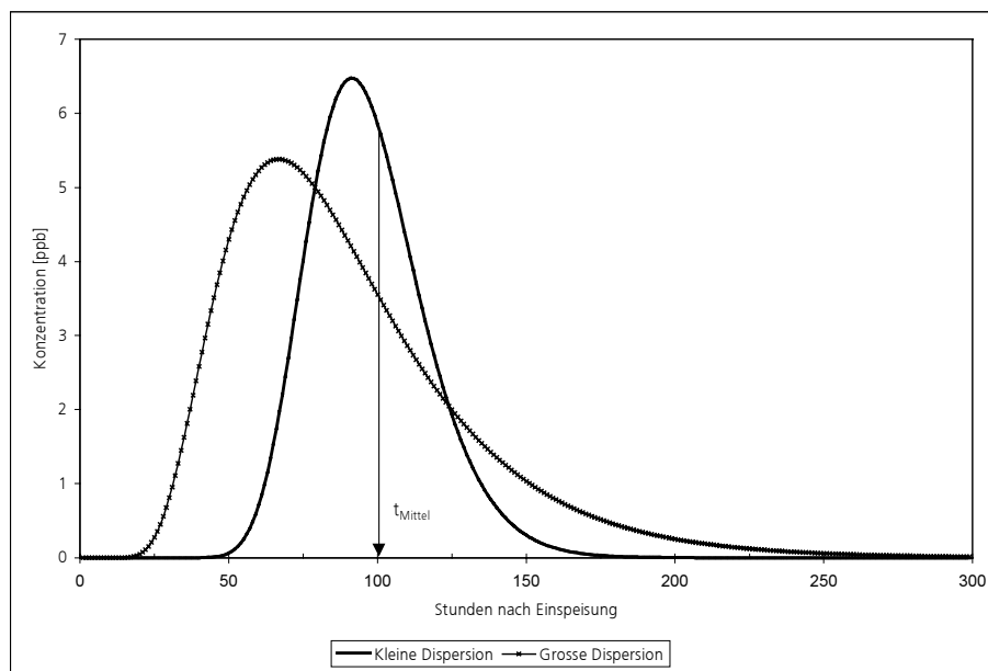
Abbildung 3.5: Zwei Tracerdurchgangskurven mit identischer mittlerer Fließzeit t_{\text{Mittel}} , aber unterschiedlich grossen Dispersionskoeffizienten.
